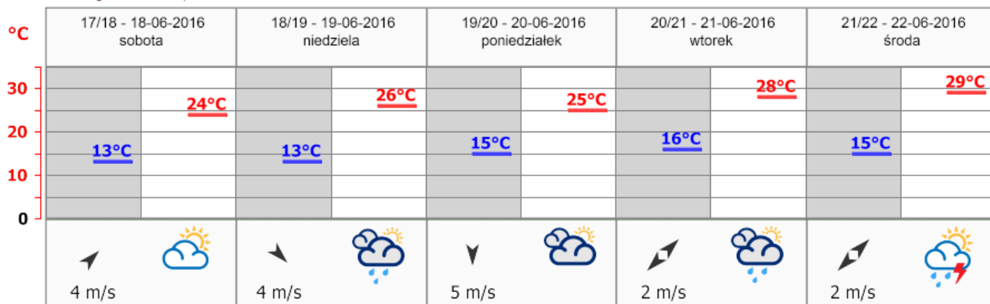
Meteogram dla Opola
